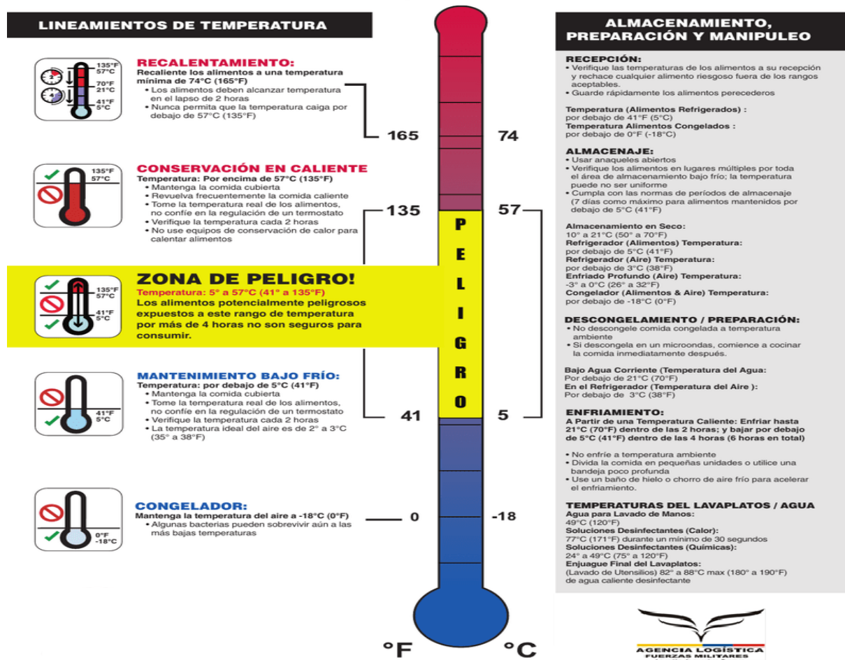
Imagen 34. Diagrama de temperatura
