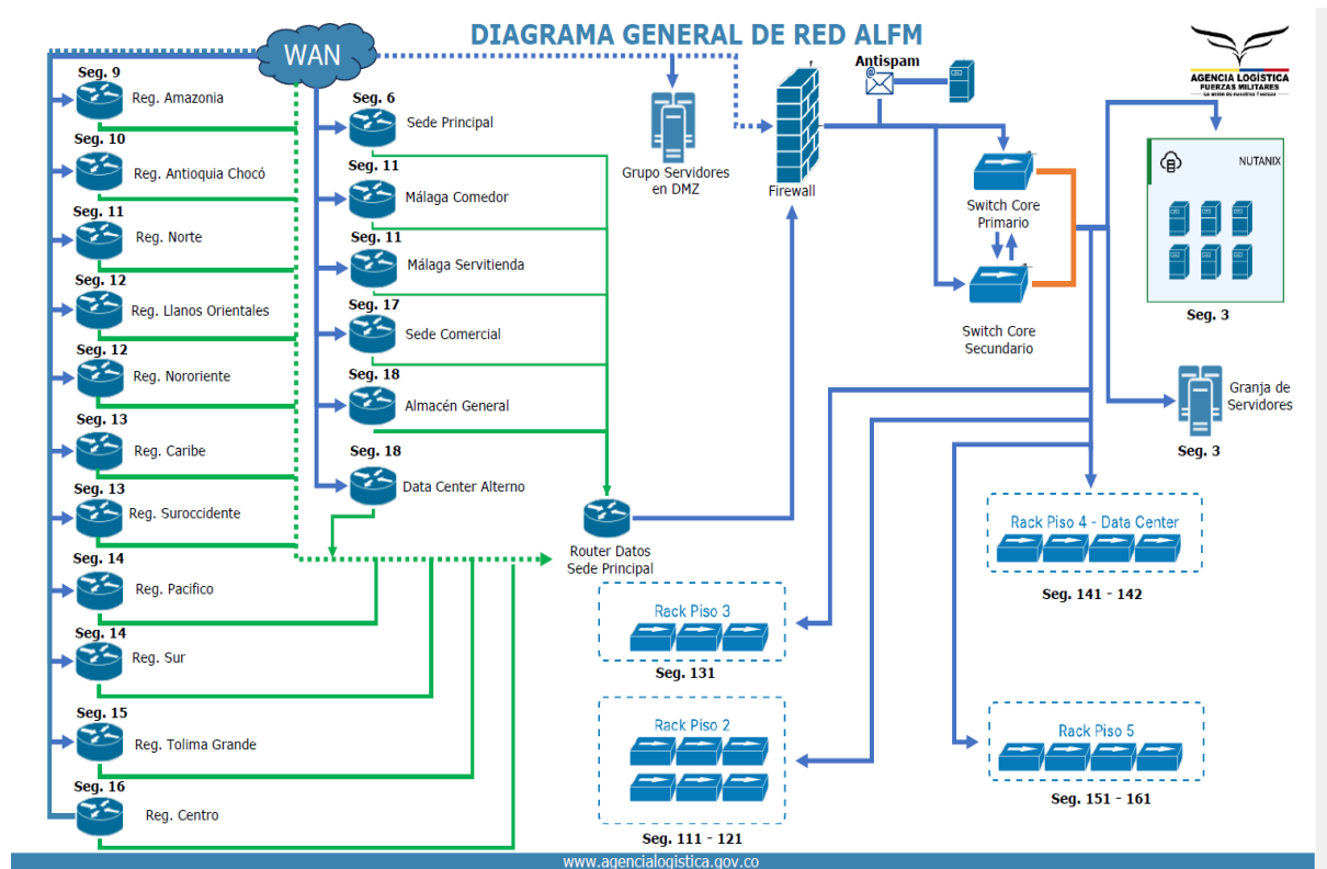
Figura 16. Topología de red local.
