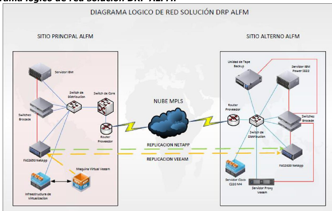
Figura 20. Diagrama lógico de red solución DRP ALFM.
