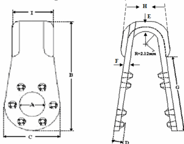
Figura 1 Gancho Rápido
