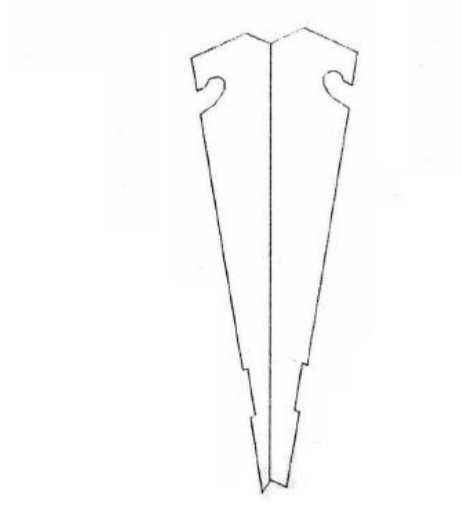
Figura 2 Detalle general de Estacas :
