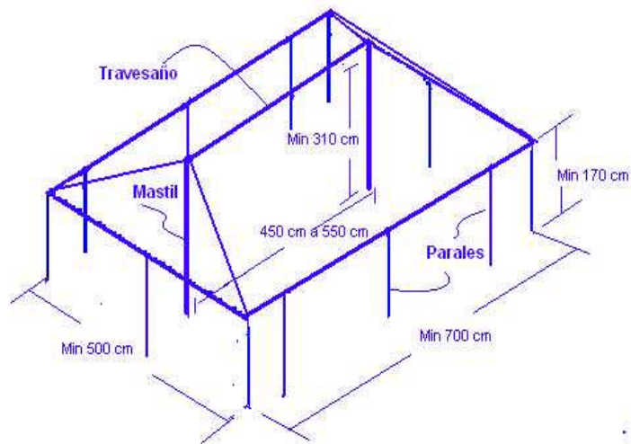
Figura 1. Detalle general de la carpa
